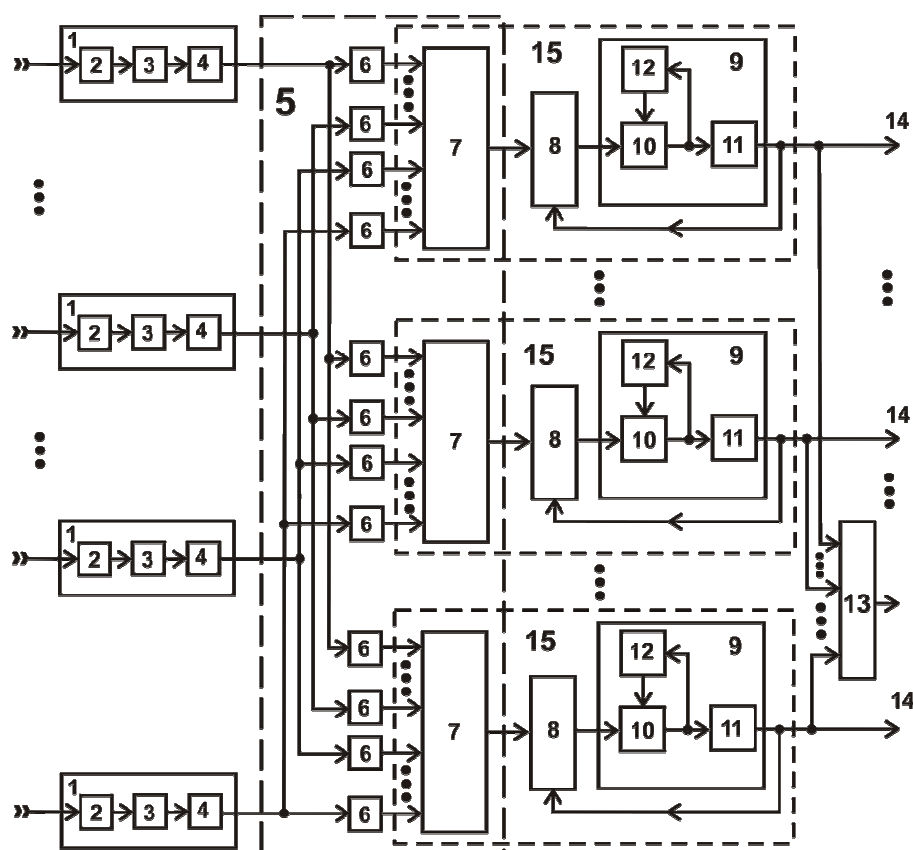
Рис. 7. Аксо-соматический нейропроцессор по а. с. 1306368 [9] содержит n блоков 1 моделирования синапса, каждый из которых состоит из согласующих элементов 2, масштабирующих коэффициентов 3 и элементов задержки 4; блок 5 моделирования аксона, в который входят весовые элементы 6 и входные сумматоры 7; m блоков 8 вызванных постсинаптических потенциалов; m формирователей 9 спайка, каждый из которых состоит из элемента сравнения 10, формирователя импульсов 11 и формирователя 12 порогового значения, выходной сумматор 13, выход которого является аксонным выходом 14. Соответствующие блоки 7-9 образуют m узлов возбуждения 15, а блок 8 выполнен в виде управляемого интегратора.
