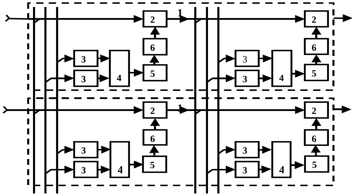
Рис. 6. Нейристорный процессор нервного пучка волокон по а. с. 1439632 [7]: 1 – нейристоры, 2 – нейристорные ячейки, 3 – масштабирующие блоки, 5 – блоки дифференцирования, 6 – элементы задержки. Показан фрагмент сети размерностью 2 x 2.
